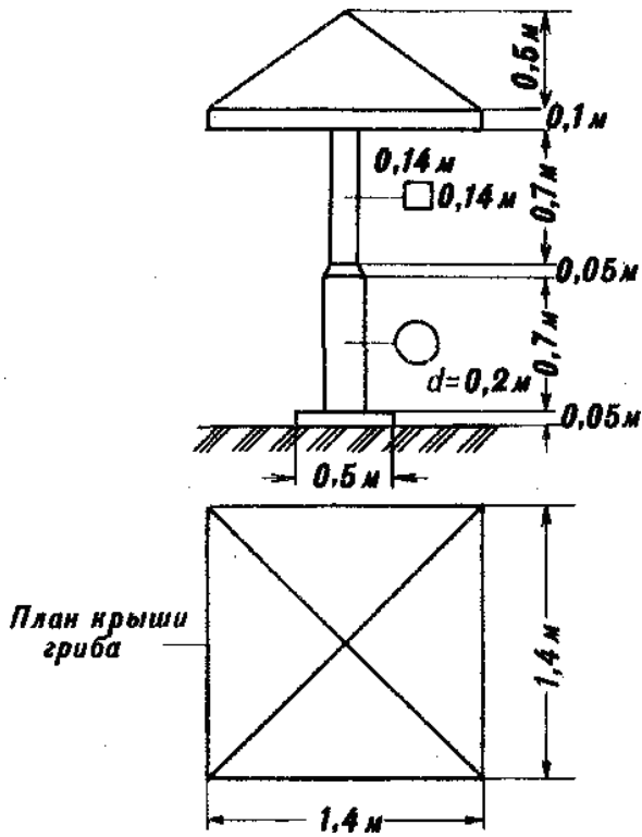
Постовой гриб
