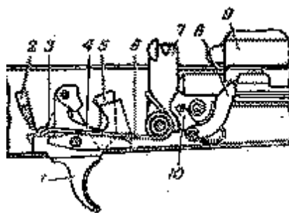
Положение частей и механизмов автомата до заряжания:
