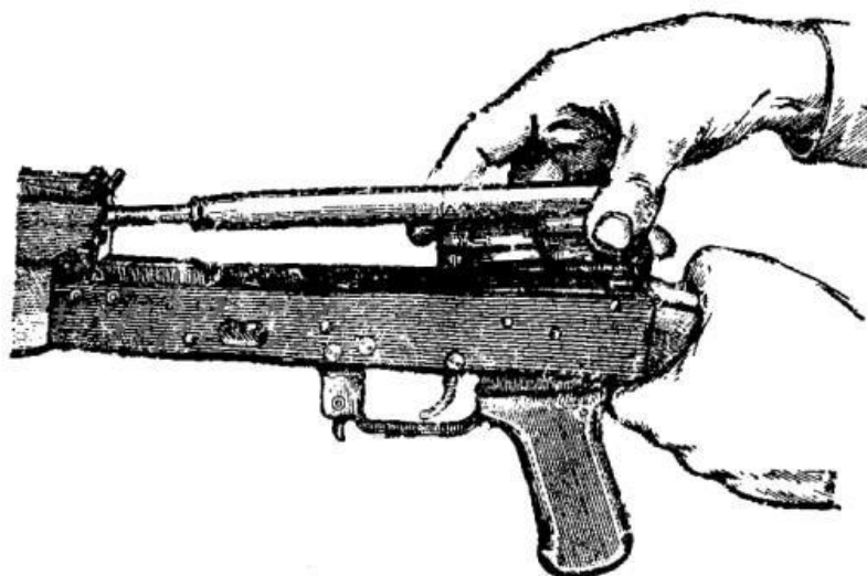
Отделение затворной рамы с затвором
