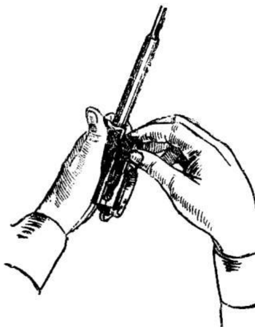
Отделение затвора от затворной рамы
