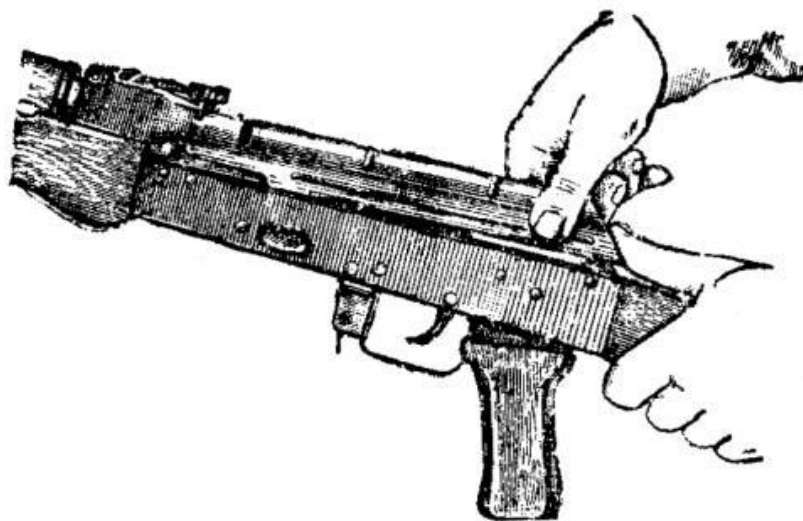
Отделение крышки ствольной коробки
