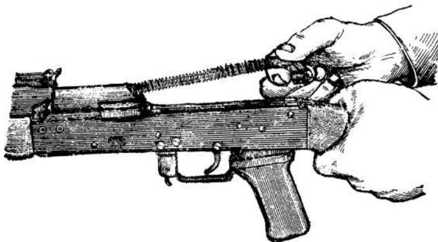
Отделение возвратного механизма
