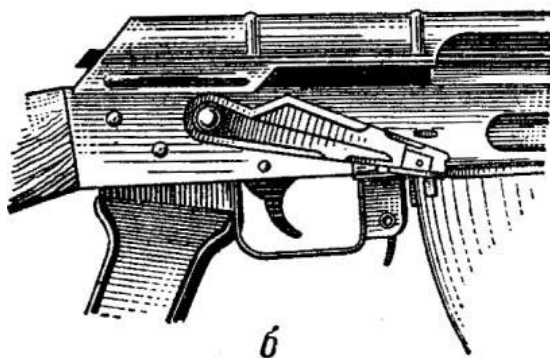
Установка переводчика на необходимый вид огня: а - для ведения автоматического огня; б - для ведения одиночного огня
