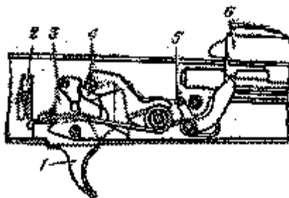
Положение частей и механизмов автомата при заряжании:
